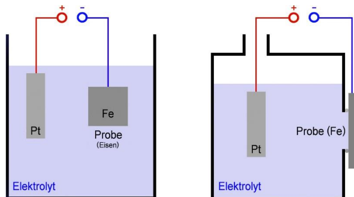
Schemata des Versuchsstands, Probe als Kathode geschaltet
